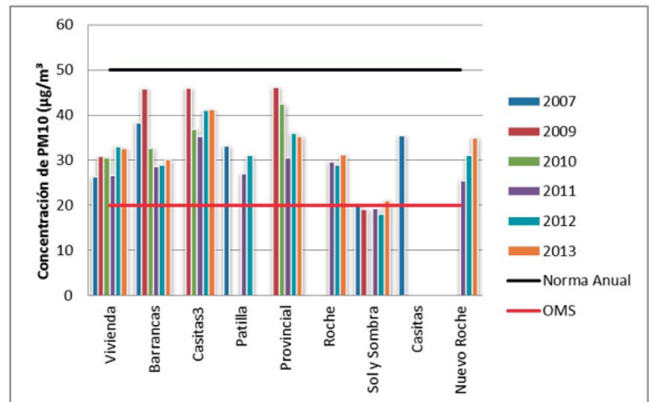
Figura 6. Promedio anual histórico de PM10 por estación.
