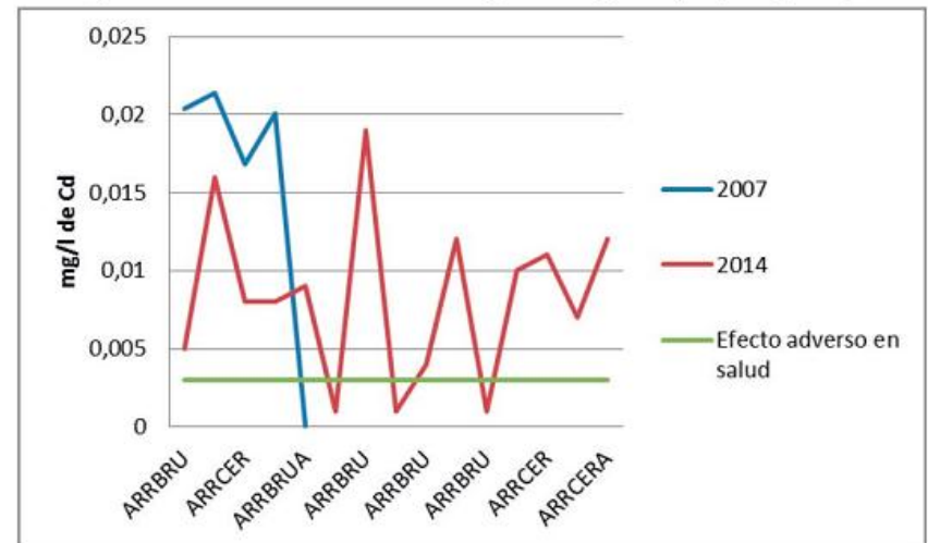
Figura 2. Concentración de cadmio arroyos Bruno y Cerrejón (2007 y 2014).
